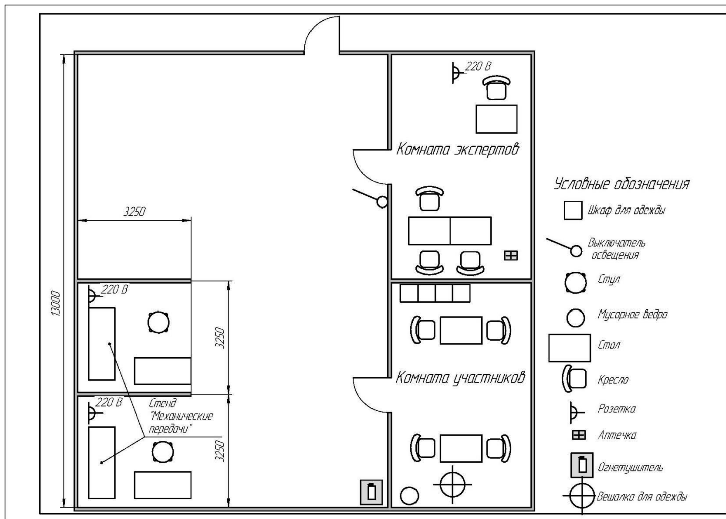
Рисунок III.1 - План застройки площадки центра проведения демонстрационного экзамена
